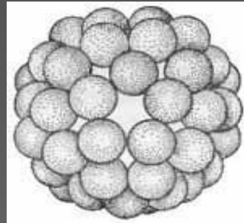
Вирус полиомиелита
