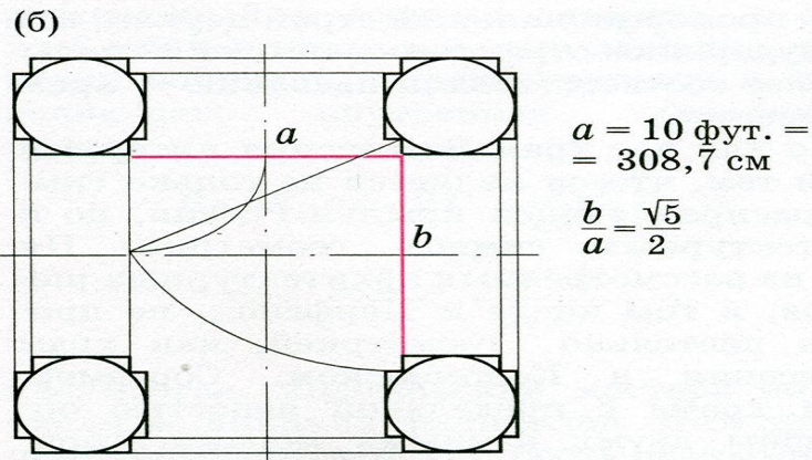
Пропорции церкви Покрова Богородицы на Нерли. Построение плана с помощью парных мер по Шевелеву (а). Геометрическое построение ядра плана по Афанасьеву (б). Некоторые пропорциональные членения западного фасада (в).
