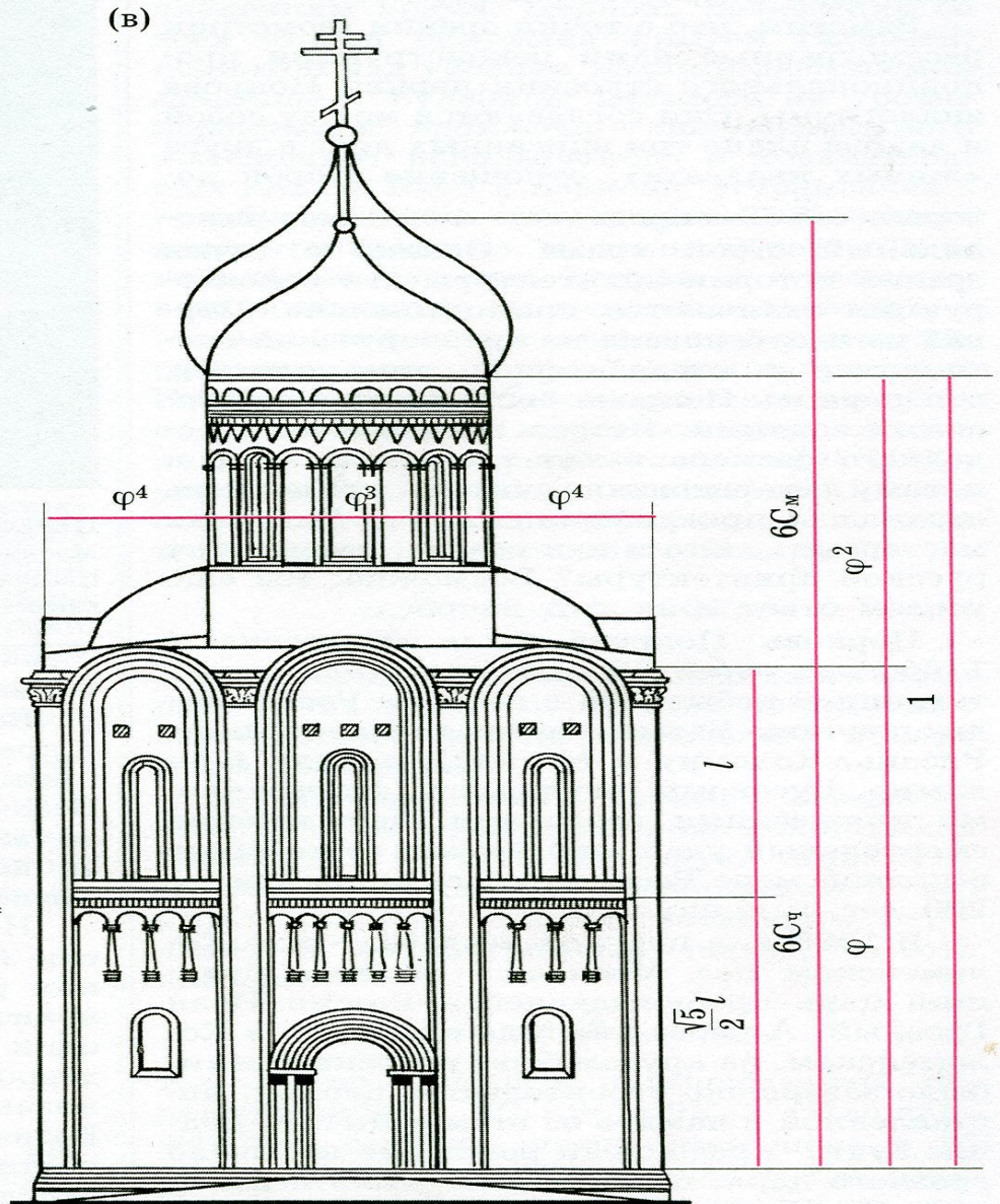
Пропорции церкви Покрова Богородицы на Нерли. Построение плана с помощью парных мер по Шевелеву (а). Геометрическое построение ядра плана по Афанасьеву (б). Некоторые пропорциональные членения западного фасада (в).
