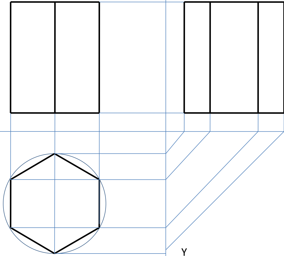
«ТРИ ВИДА» шестиугольной прямой призмы
