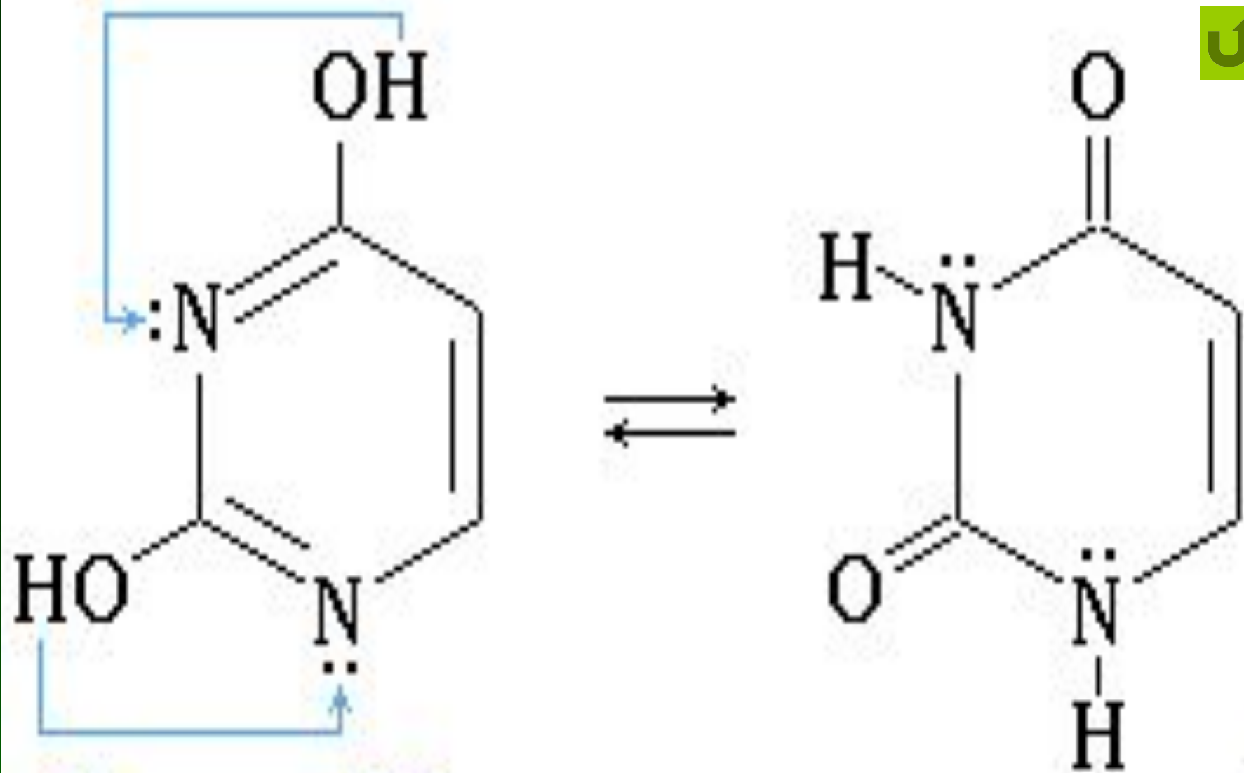
Урацил (2,4-дигидроксиимидин)
