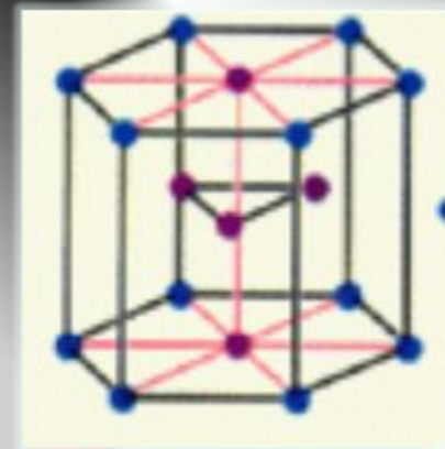
Гексагональная
