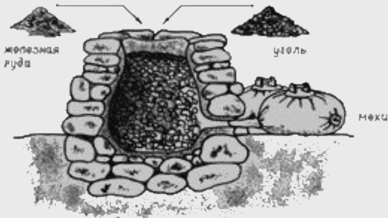
Получение губчатого железа в каменном горне
