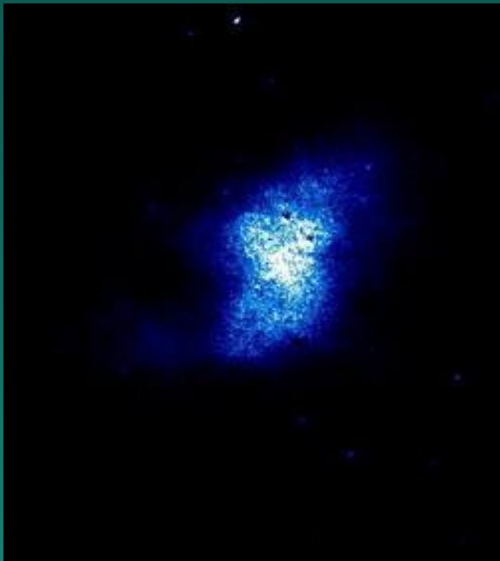
Рентгеновское излучение
