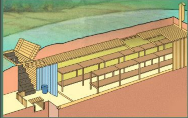
Противорадиационное укрытие
