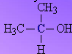
вторичный пропанол
