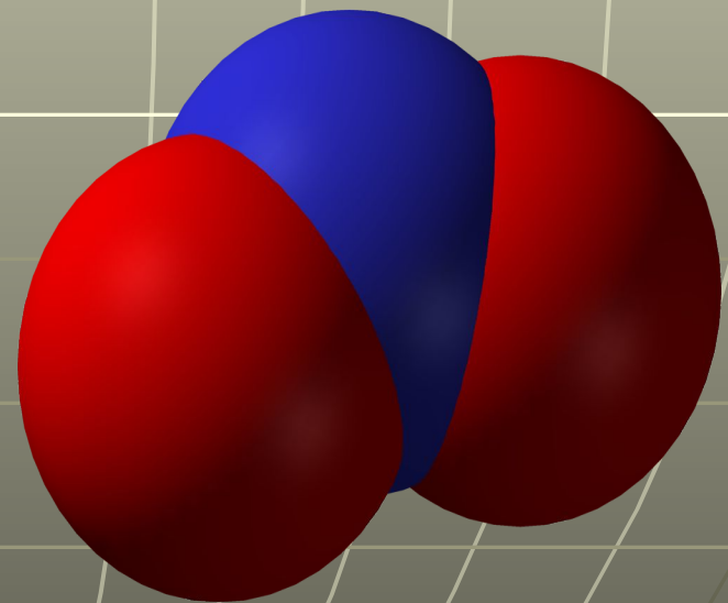
Оксид азота IV
