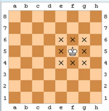
Ход короля
