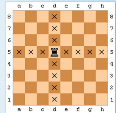
Ход ладьи
