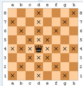
Ход ферзя
