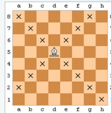
Ход слона
