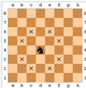
Ход коня
