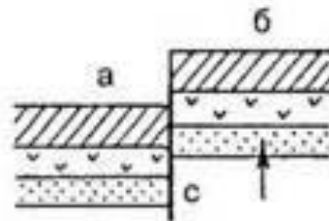
Взброс
