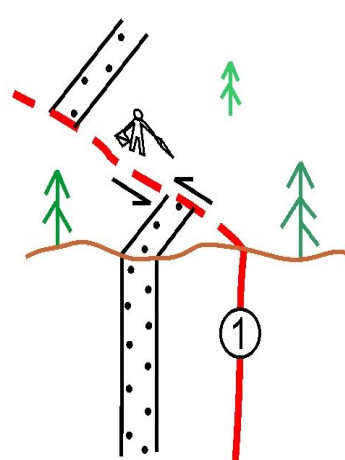
ЛЕВЫЙ СДВИГ
