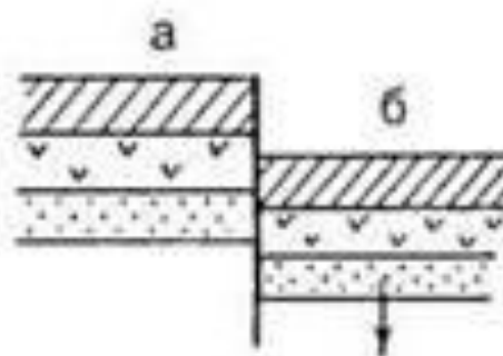
Сброс
