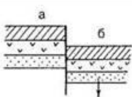
Сброс
