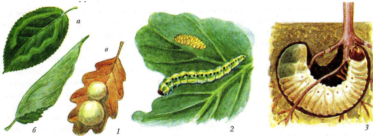
Рис. 1: 1 – типы повреждений растений насекомыми ( a – «минирование», б – свертывание, в – галлы); 2 – кладка и личинки бабочки-капустницы на листьях; 3 – личинки майского хруща (в почве вблизи корней)
