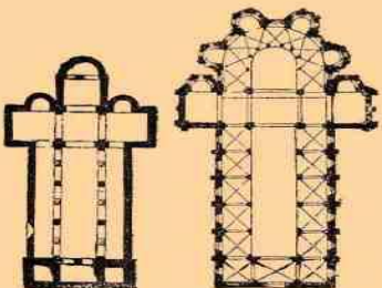
1. Геклингенская церковь (план). 2. Церковь Notre Dame du Port в Клермонте (план).
