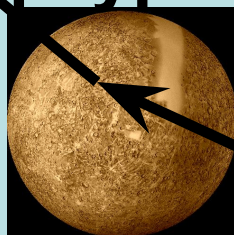
Меркурий
