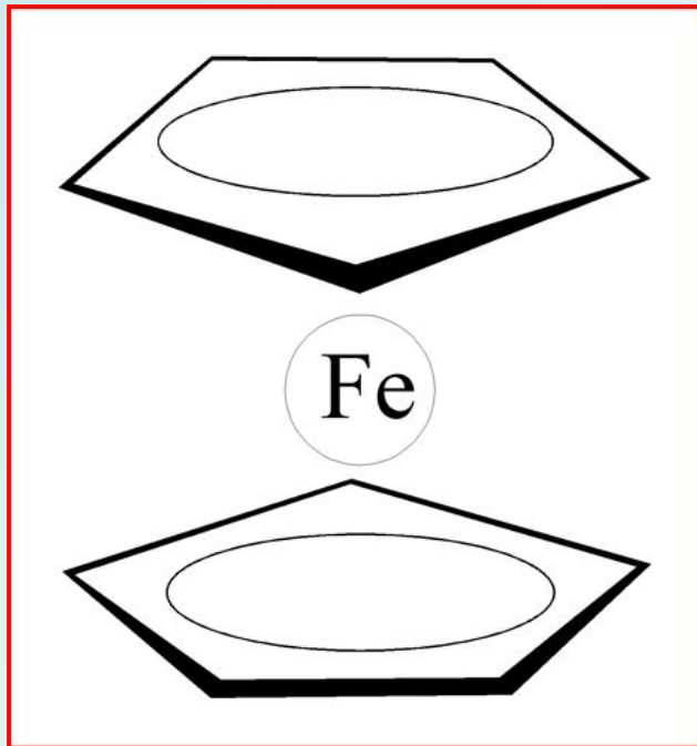
Дициклопентадиенилжелезо
