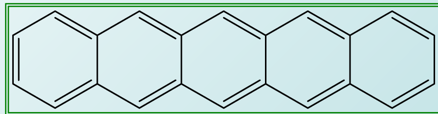
Пентацен
