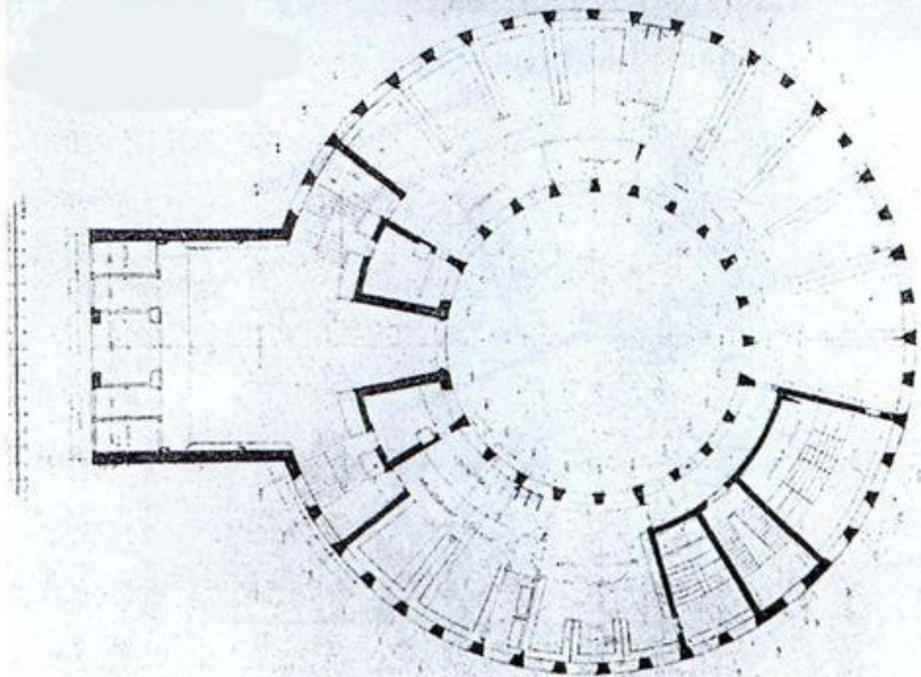
Круглая баня. План
