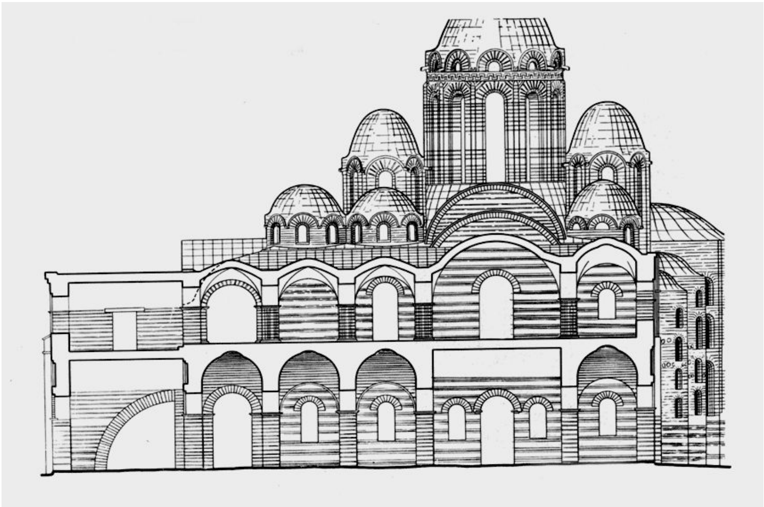
Продольный разрез
