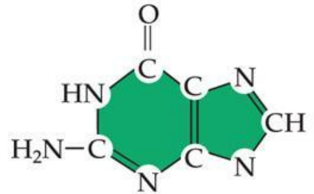
Гуанин, Г
