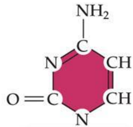
Цитозин, Ц
