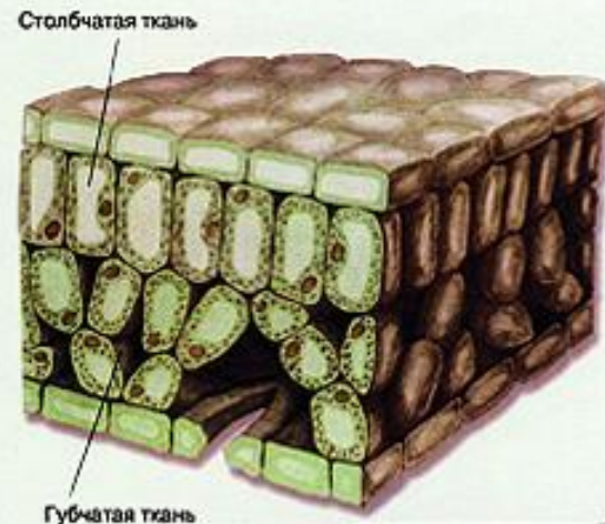
ОСНОВНАЯ ТКАНЬ
