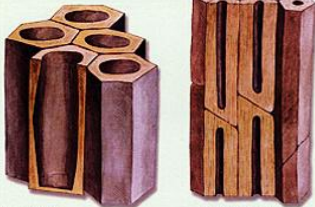
МЕХАНИЧЕСКАЯ ТКАНЬ
