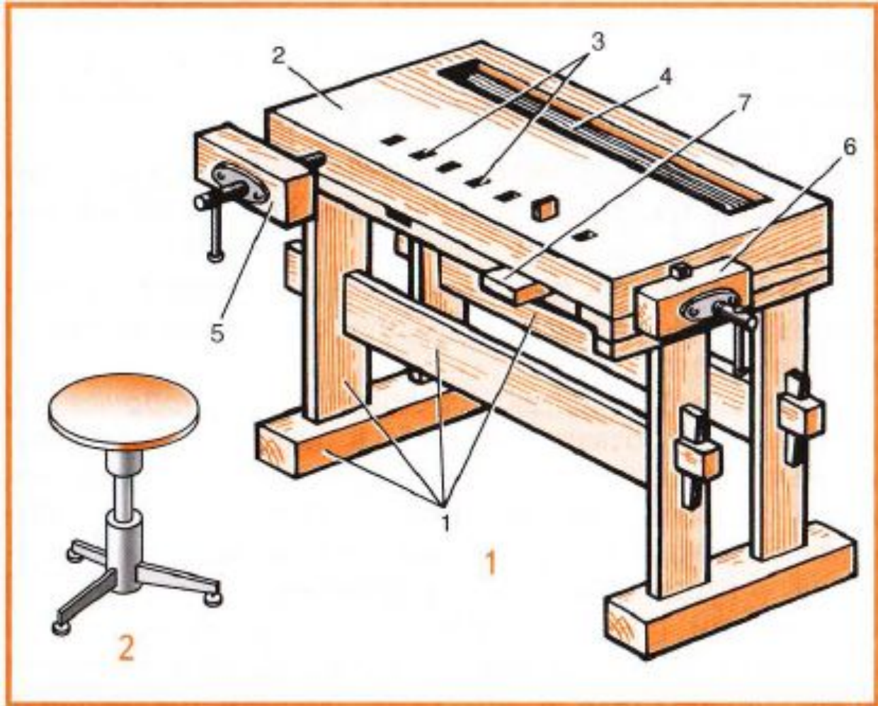
Рис 1. Столярный верстак
