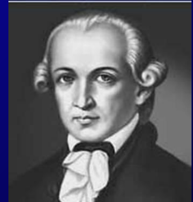
Иммануил Кант
