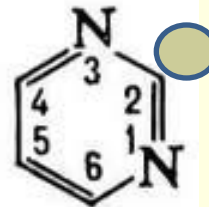
Пиримидин
