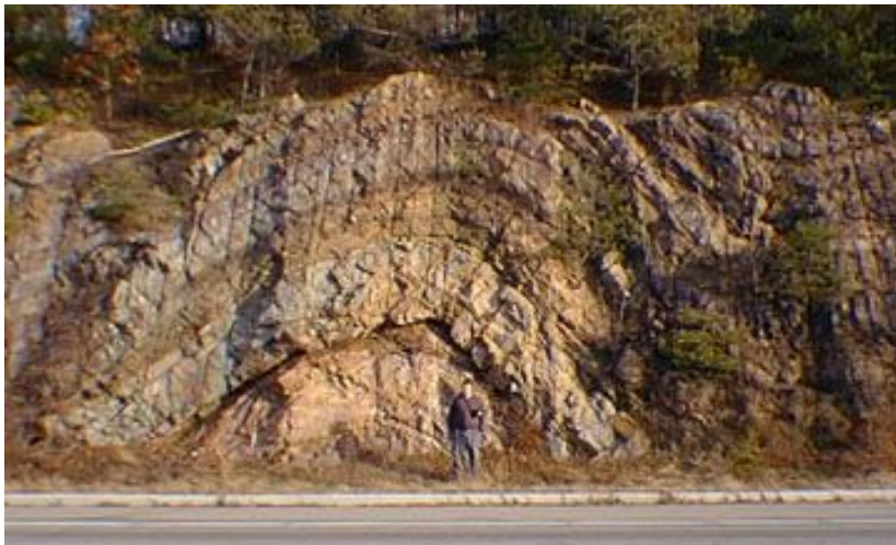
антиклинальная складка
