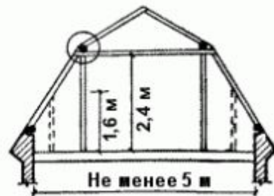
Полувальмовые
