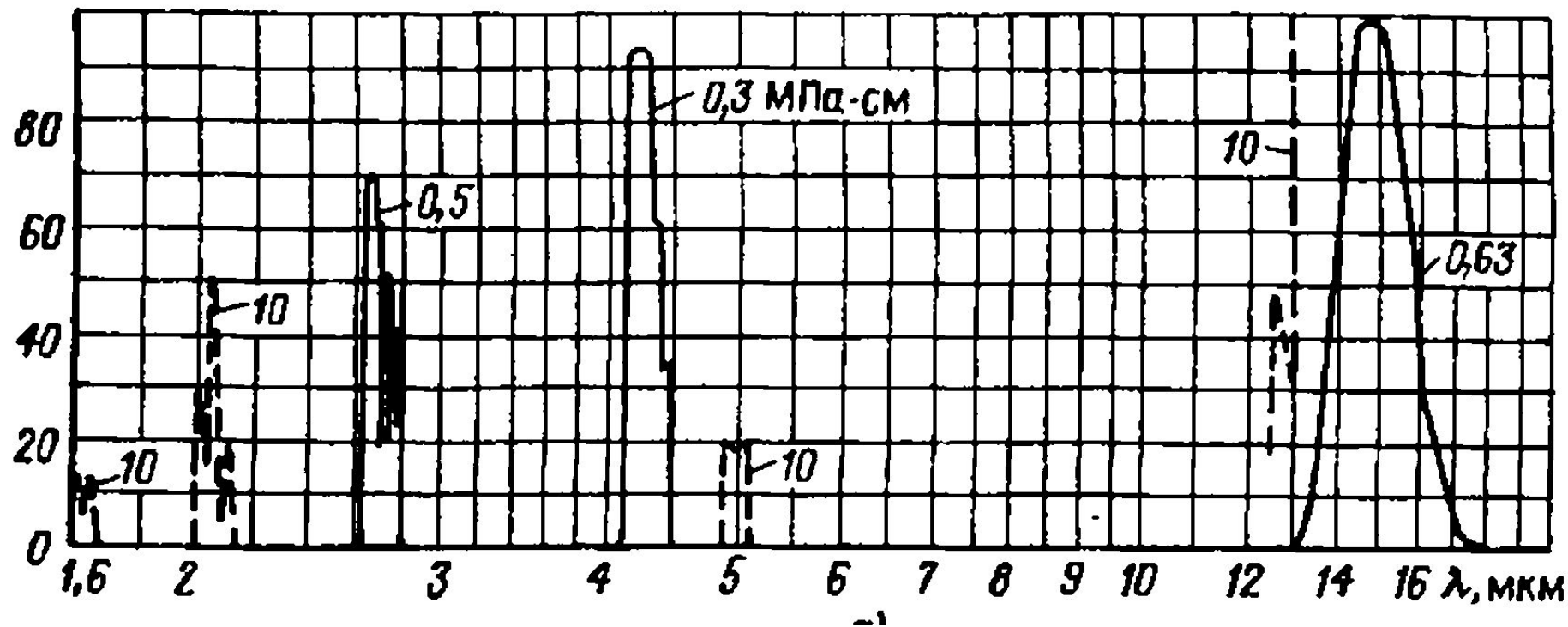
Спектр поглощения углекислого газа [1]
