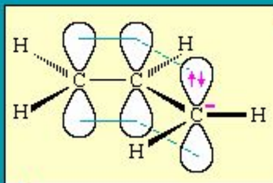
\text{CH}_2=\text{CH}-\overset{-}{\text{C}}\text{H}_2 аллил-анион
