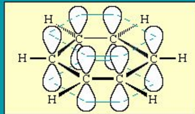
\text{C}_6\text{H}_6 бензол
