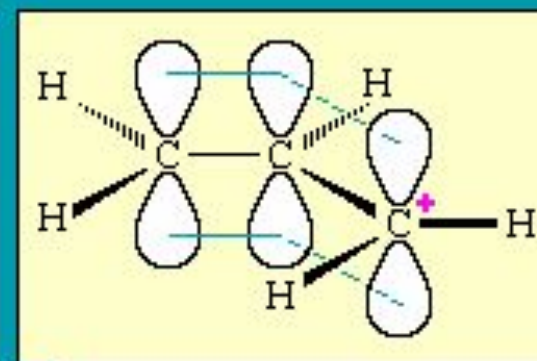
\text{CH}_2=\text{CH}-\overset{+}{\text{C}}\text{H}_2 аллил-катион
