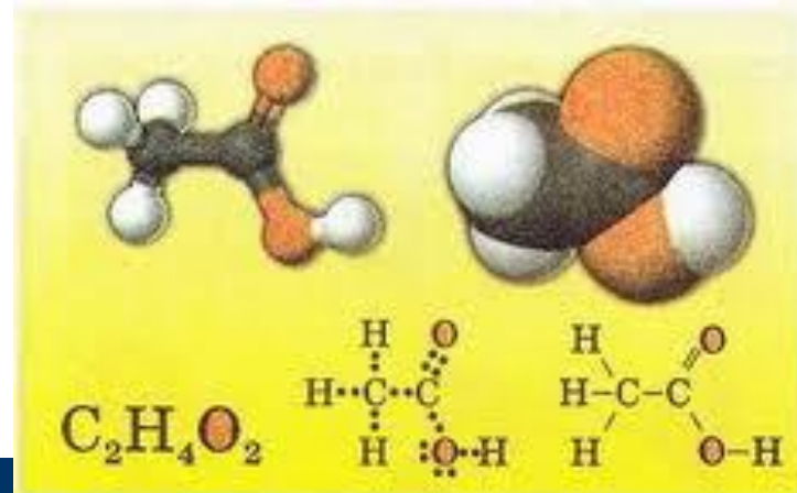
Мал. 29.1. Кулестержнева й масштабна моделі молекули оцтової кислоти, її молекулярна, електронна та структурна формули
