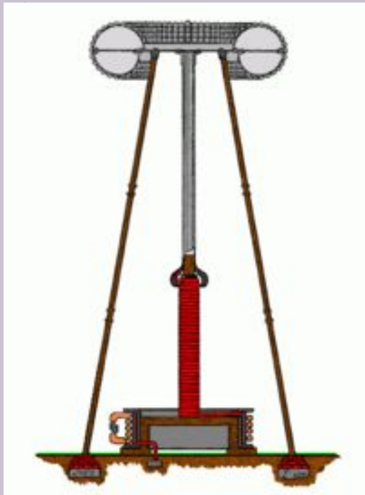
Трансформатор Тесли
