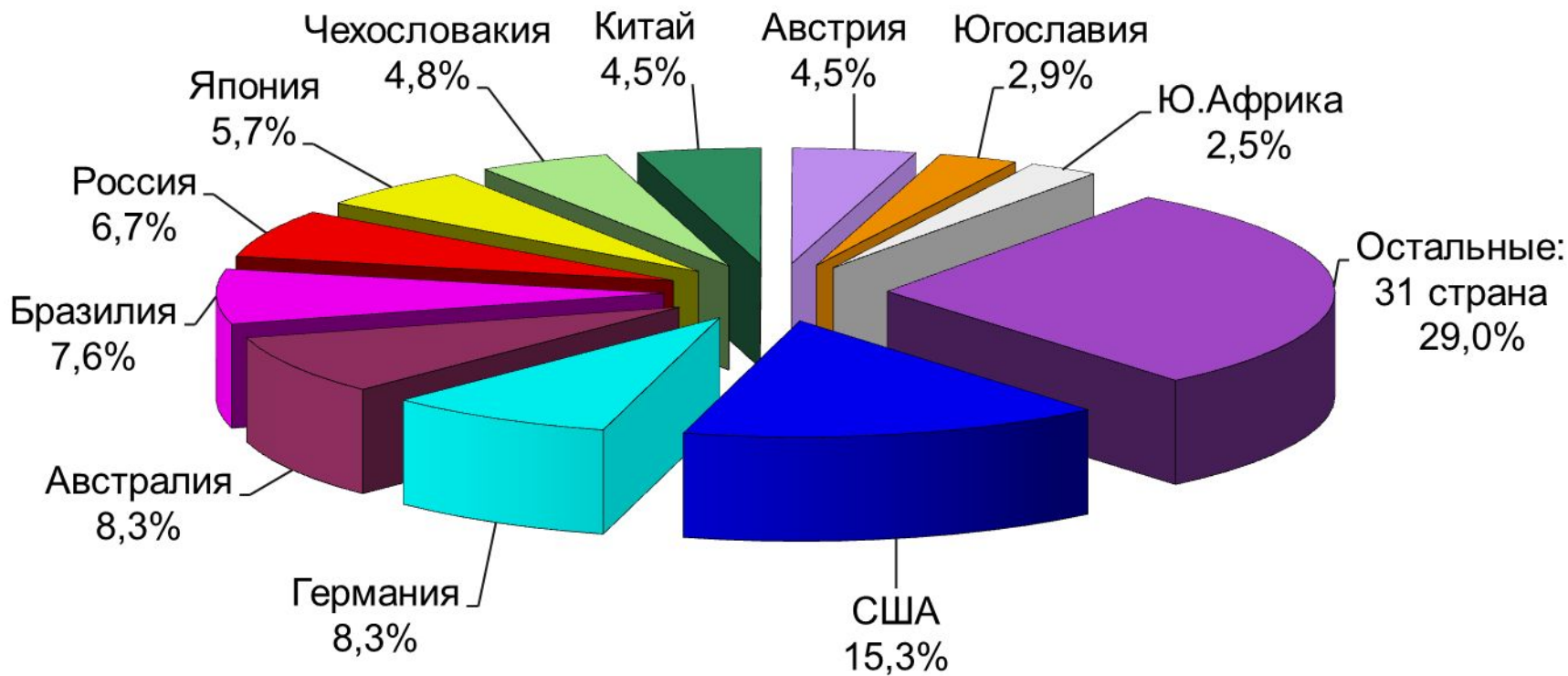
Рис.2 Вклад основных стран в публикации по производству ^{99}\text{Mo} и ^{99\text{m}}\text{Tc} для ядерной медицины (БД INIS)
