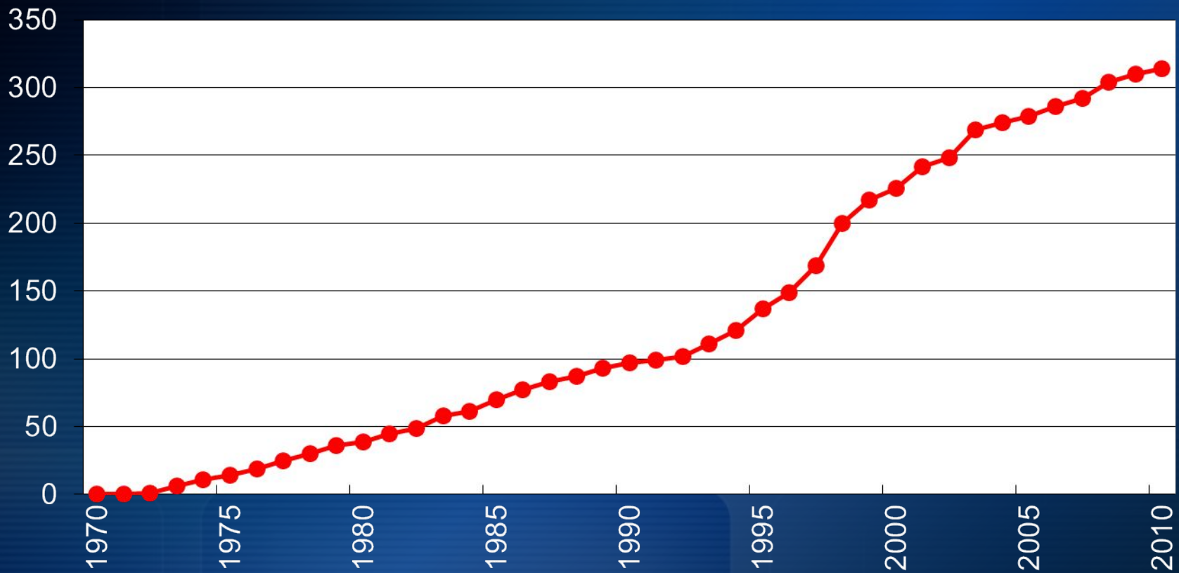
Рис.1 Динамика информационного потока по производству ^{99}\text{Mo} и ^{99\text{m}}\text{Tc} для ядерной медицины (БД INIS)
