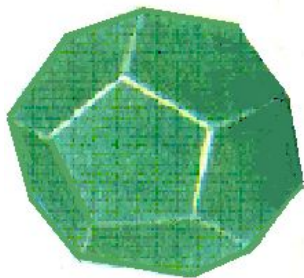
Правильный додекаэдр
