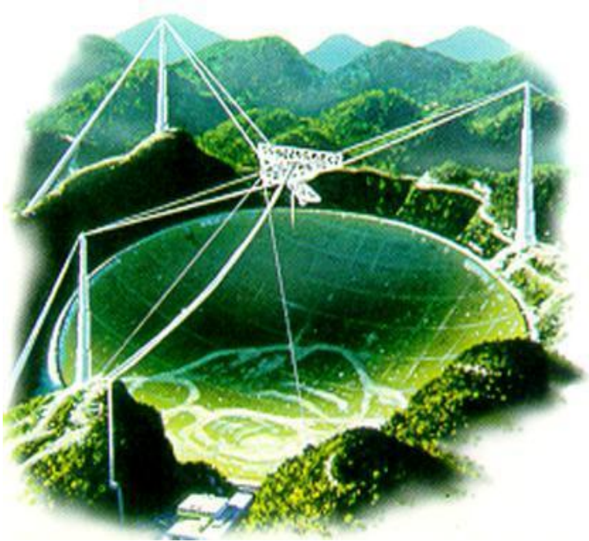
Радиотелескоп в Аресибо Пуэрто-Рико
