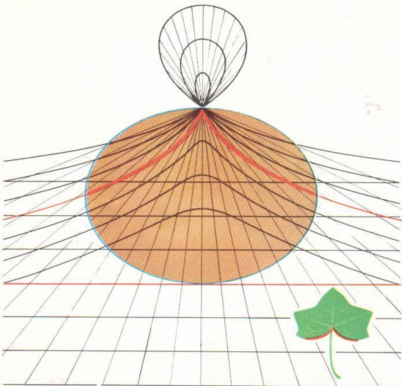
Здесь изображено семейство замечательных кривых — циссоид. Мы взяли циссоиду, рассмотрев тот участок циссоиды, который рассмат-
