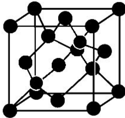
б ● Углерод
