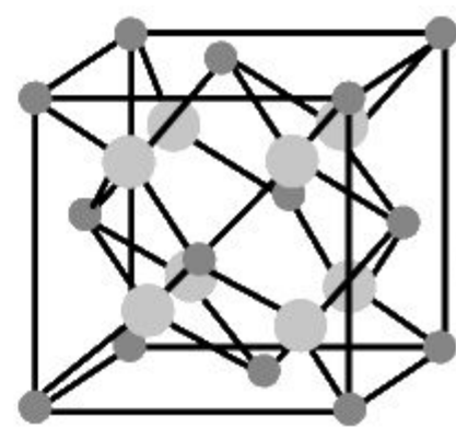
в ● Кальций ● Фтор
