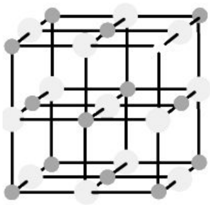
a ● Натрий ● Хлор
