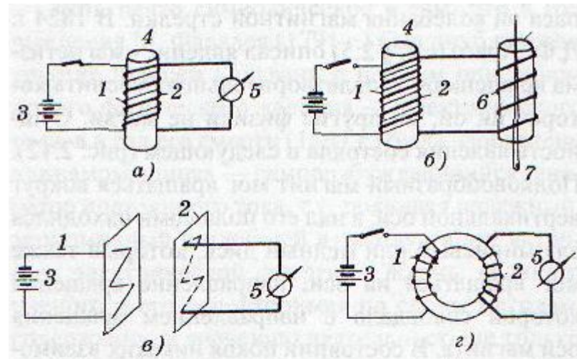
Схемы основных опытов, в результате которых было открыто явление электромагнитной индукции
