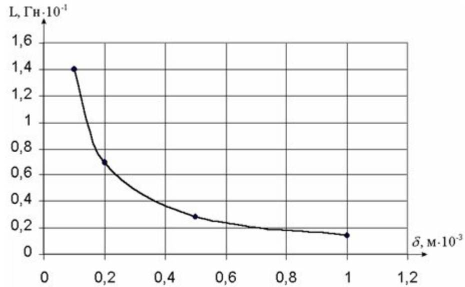
Статическая характеристика индуктивного датчика
