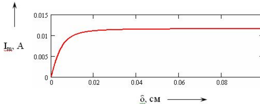
Характеристика управления индуктивного датчика
