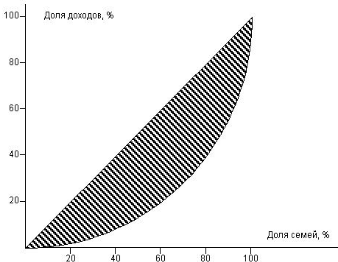
Кривая Лоренца
