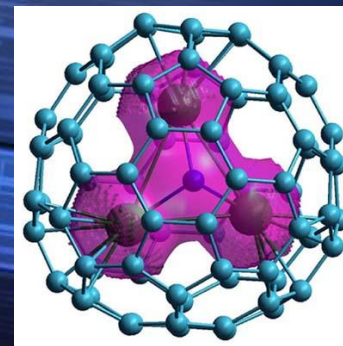
Фуллерен
