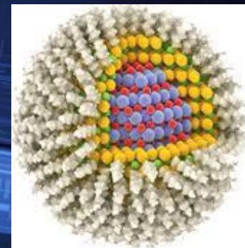
Квантовая точка
