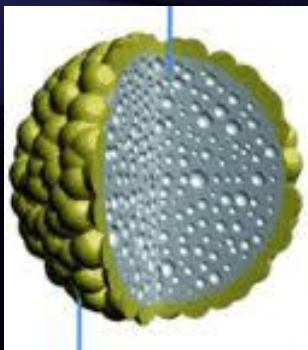
Нанооболочки
