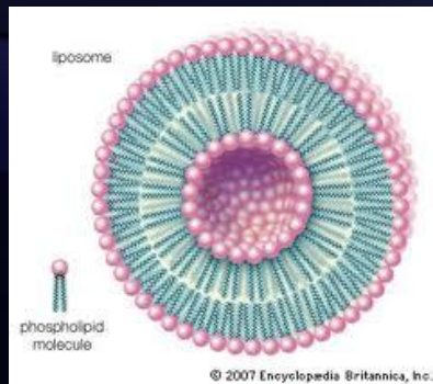
Липосома
