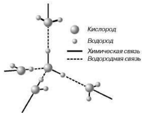
Рис. 1.6. Схема объединения молекул воды
