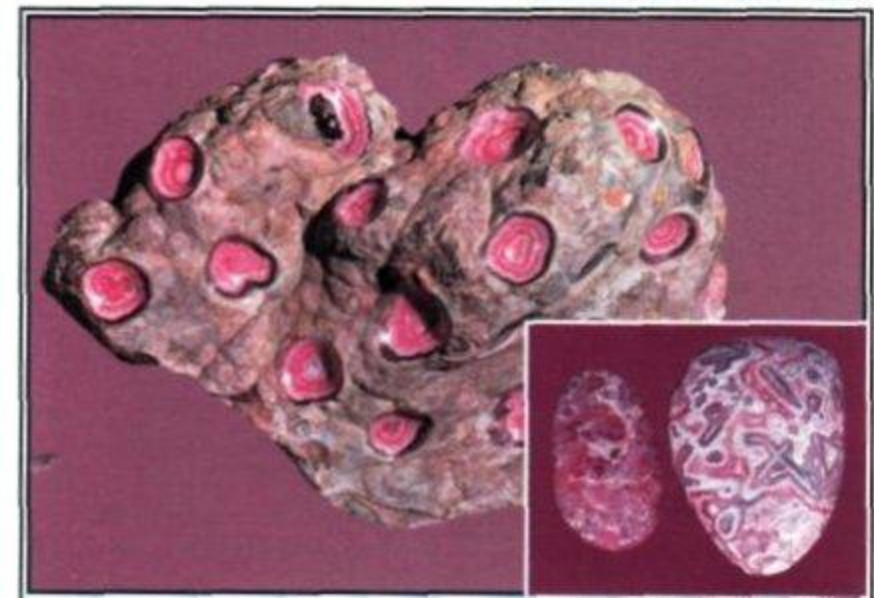
Родохрозит
