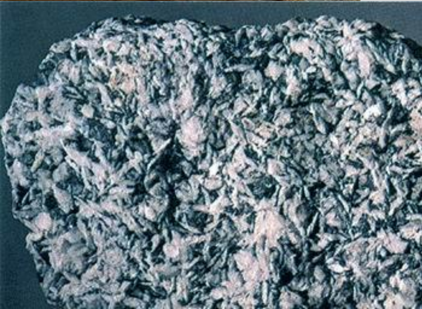
Магнезит
