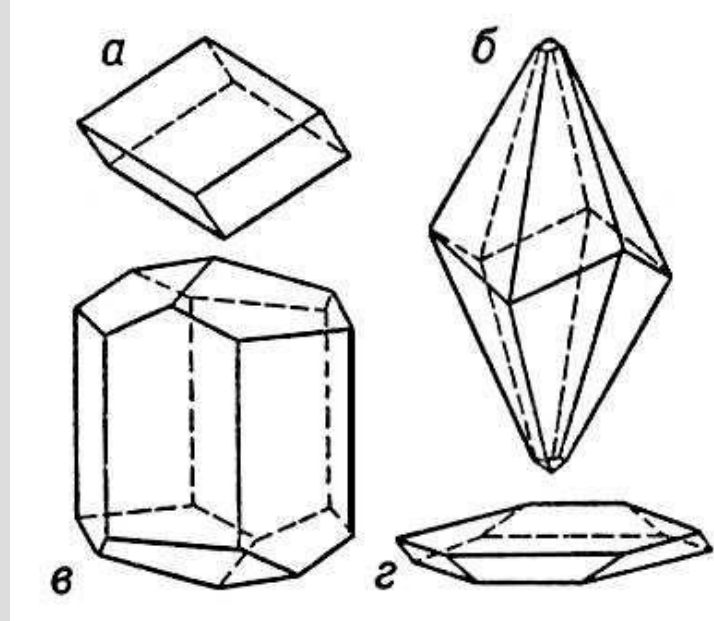
Кальцит
