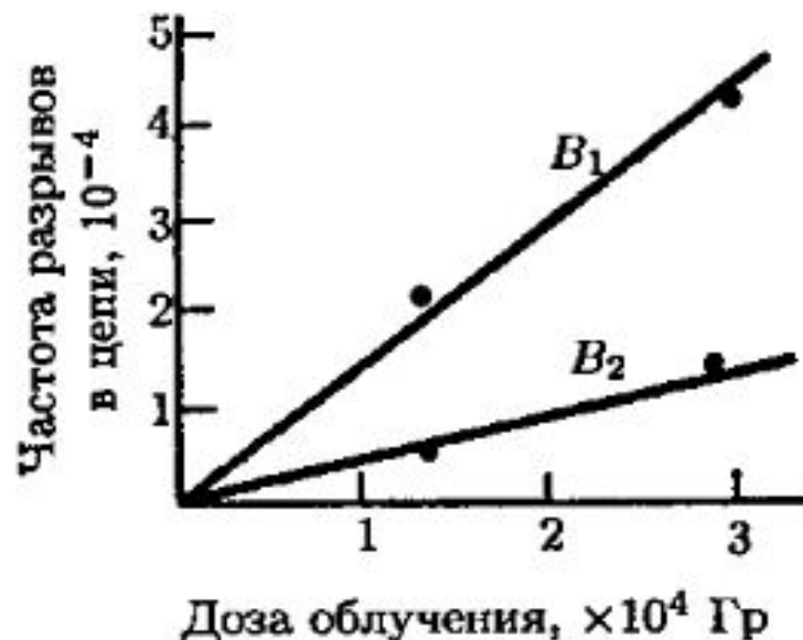
Рис. IV.13. Зависимость образования однонитевых ( B_1 ) и двунитевых ( B_2 ) разрывов в сухой ДНК тимуса теленка от дозы рентгеновского облучения в вакууме
