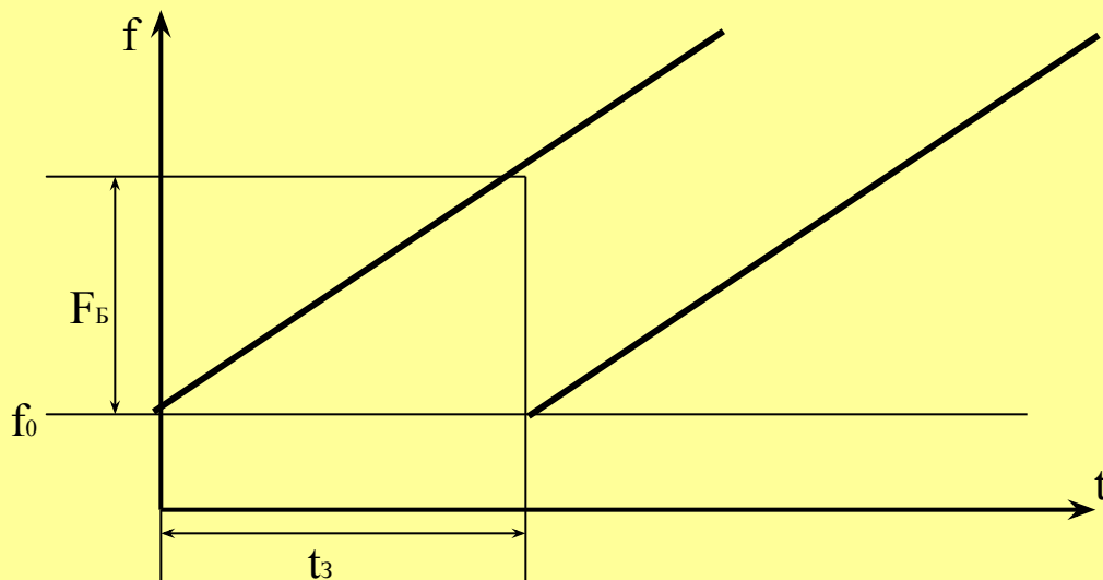
Рис. 9. Часові діаграми до структурної схеми частотної РЛС
