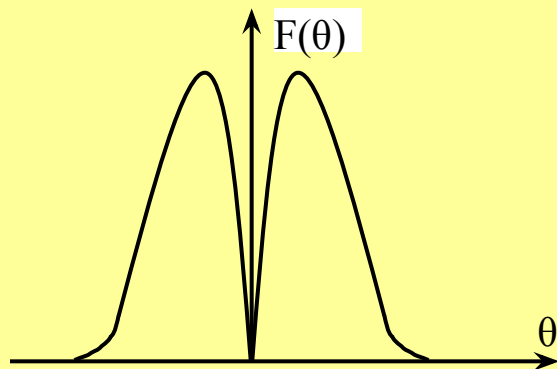
Рис. 13. ПХ для методу мінімуму
