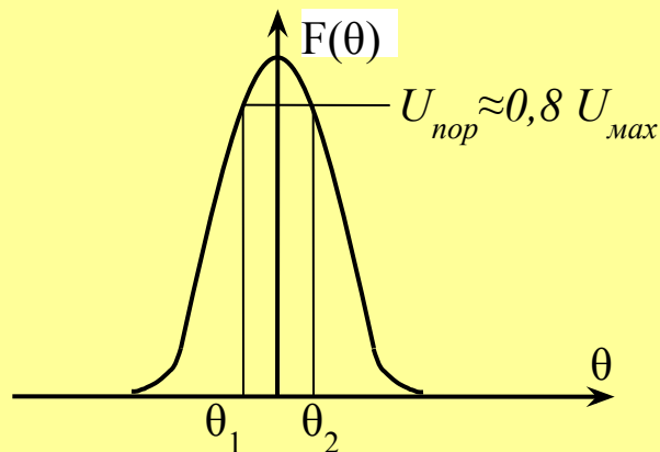
Рис. 14. ПХ для методу порівняння
