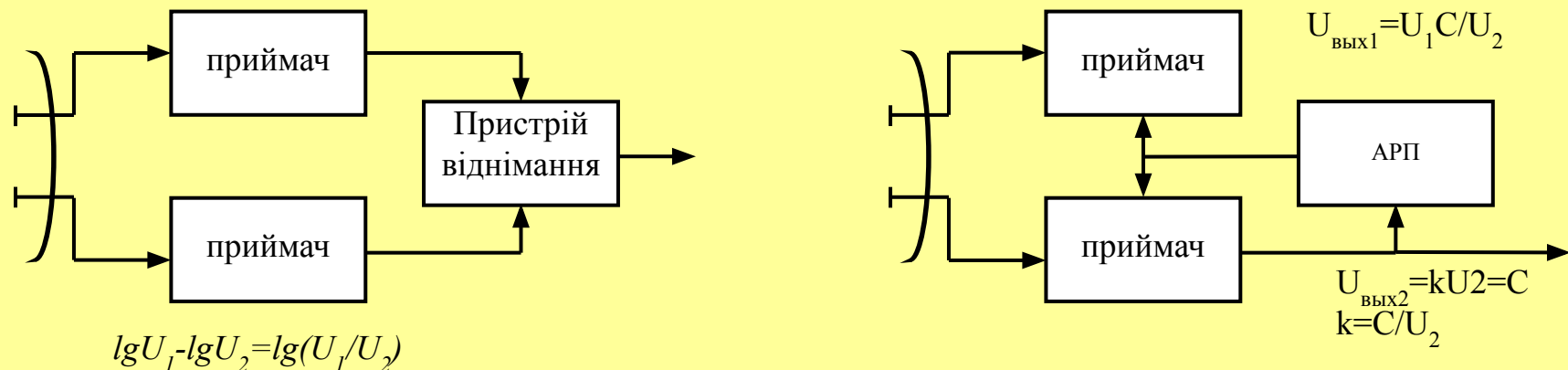
Рис. 18. Структурні схеми побудови МАП
