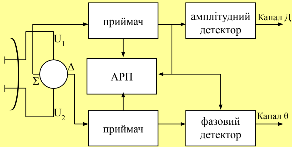
Рис. 19. Структурна схема МАП з сумарно-різницевою обробкою сигналів
