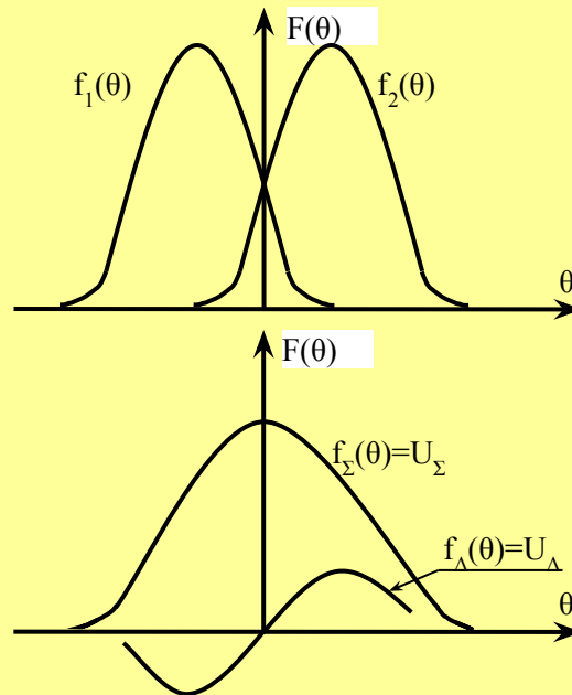
Рис. 20. ДН і сумарно-різницева її характеристика
