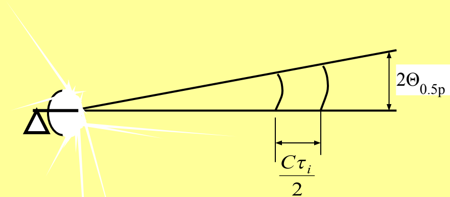
Рис. 7. Пояснення до роздільного об'єму
