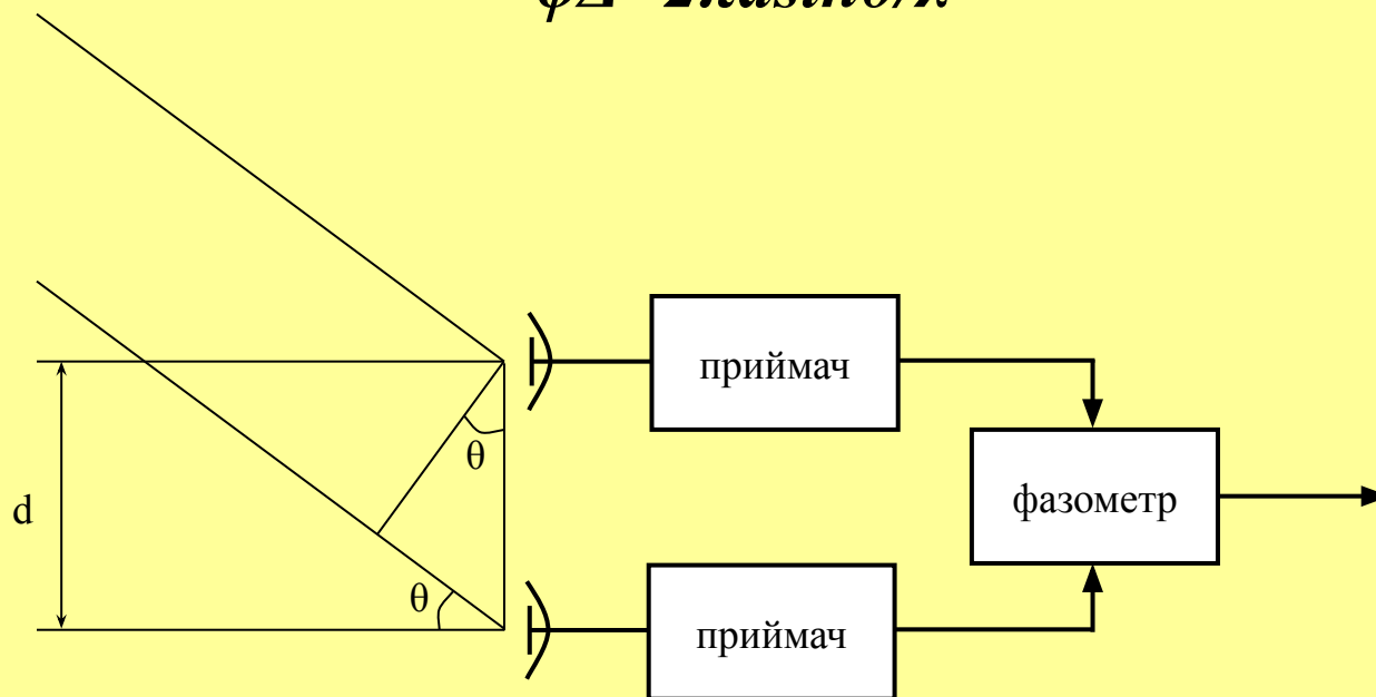
Рис. 22. Структурна схема моноімпульсного фазового пеленгатора (МФП)
