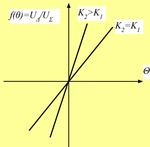
Рис. 21. ПХ сумарно-різницевого МАП
