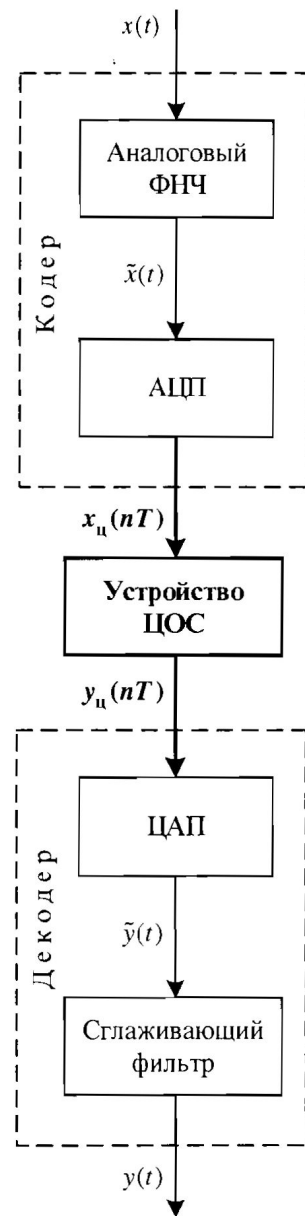
Рис. 1.1. Обобщенная схема цифровой обработки сигнала
