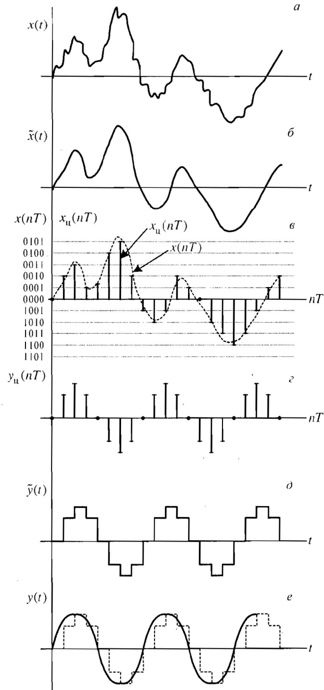
Рис. 1.1. Обобщенная схема цифровой обработки сигнала
