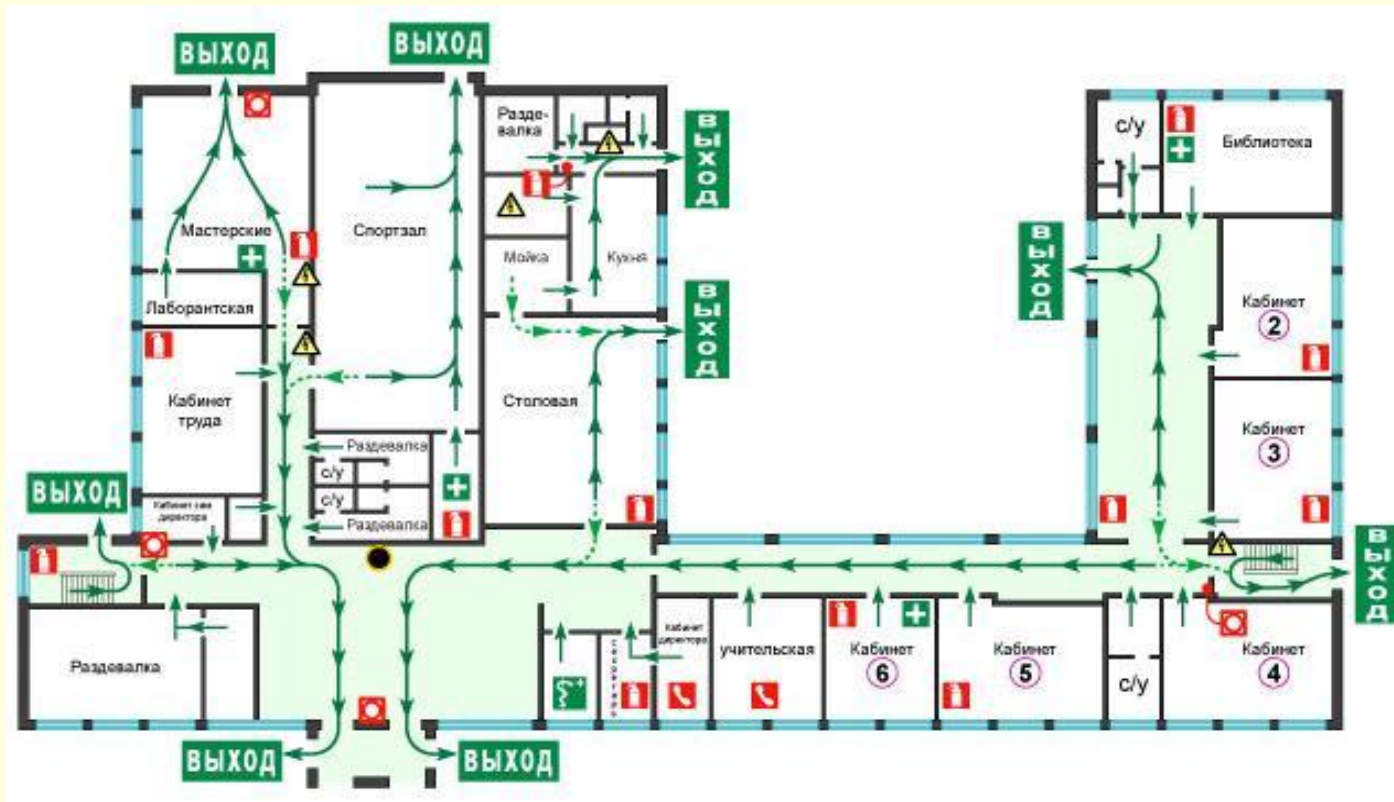
Рисунок 13 Схема эвакуации при пожаре с объекта, на котором производится работы
