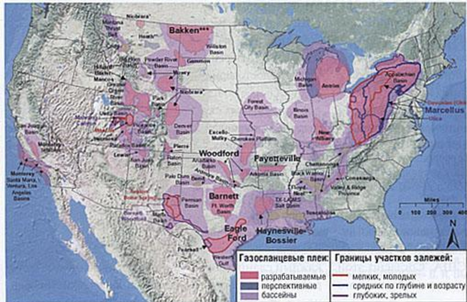
Карта газосланцевых плеев США (Источник: EIA, http://www.eia.gov/oil_gas/rpd/shale_gas.pdf )
