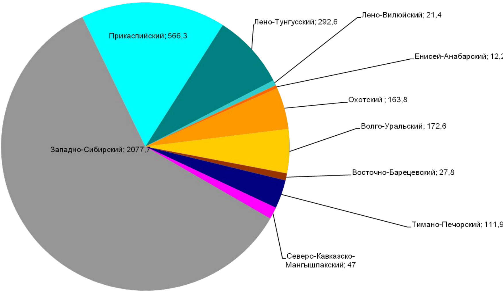
Распределение извлекаемых запасов конденсата по нефтегазоносным бассейнам Российской Федерации, млн т /Ставский и др.,2013/
