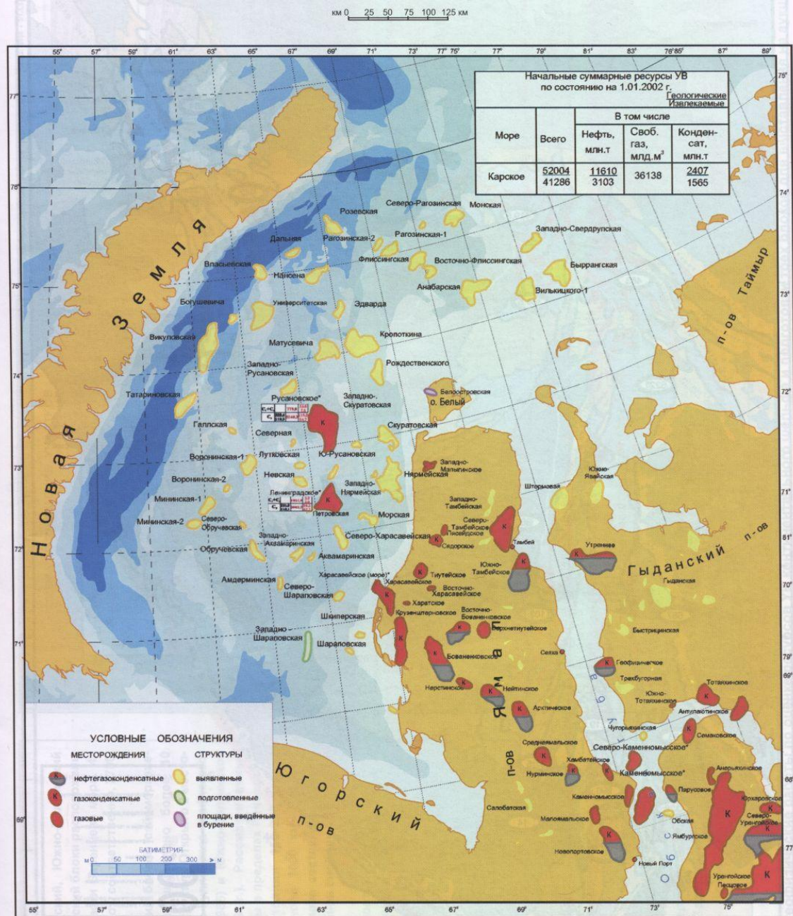
Рис. 5. Нефтегазоносный ресурсный потенциал Карского моря
