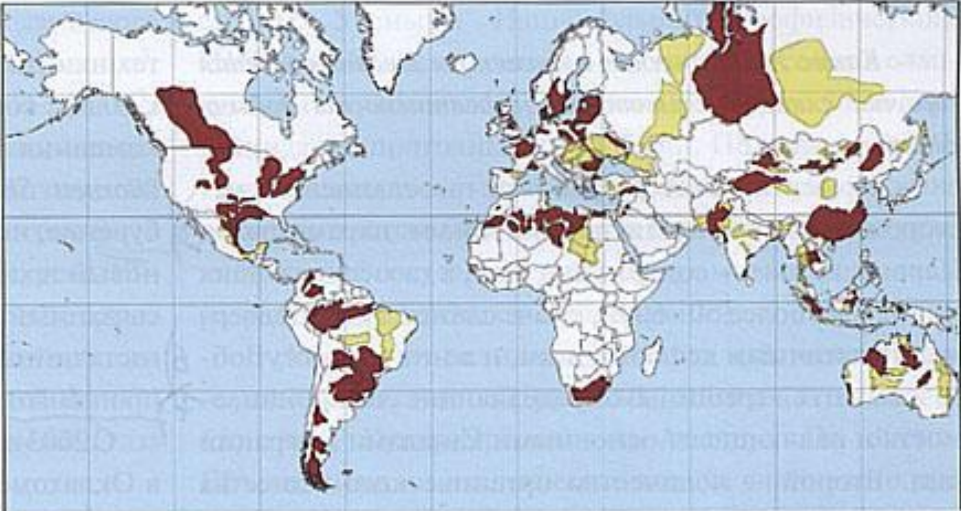
Карта размещения сланцевых формаций (по состоянию на май 2013 г.) [7]: ■ с доказанными запасами и технически извлекаемыми ресурсами нефти и газа ■ с прогнозными ресурсами нефти и газа
