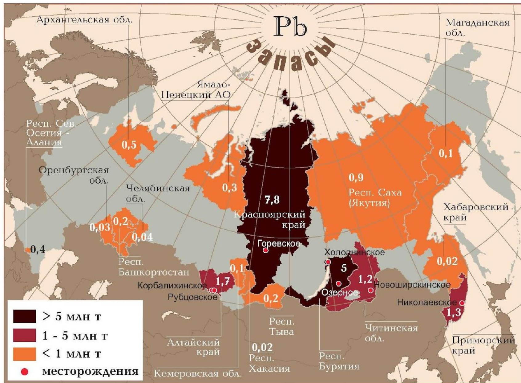
Основные месторождения свинца и распределение его балансовых запасов по субъектам РФ, млн т /Госдоклад, 2007/
