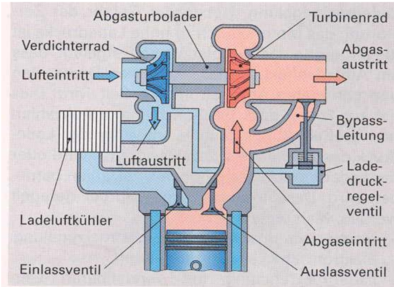
Bild 5: Schema eines Motors mit Abgasturbolader
