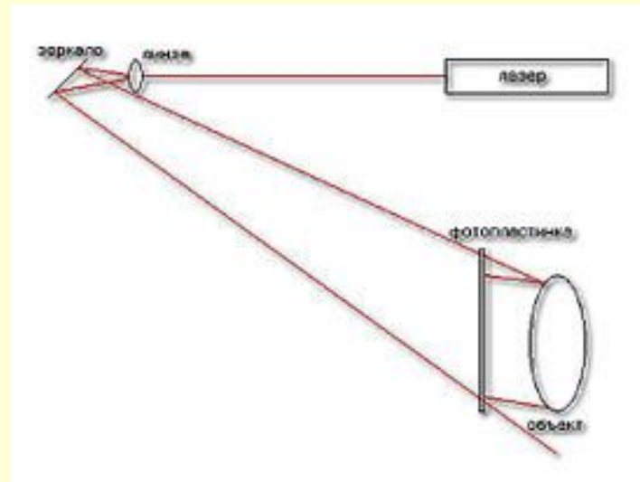
Схема Денисюка
