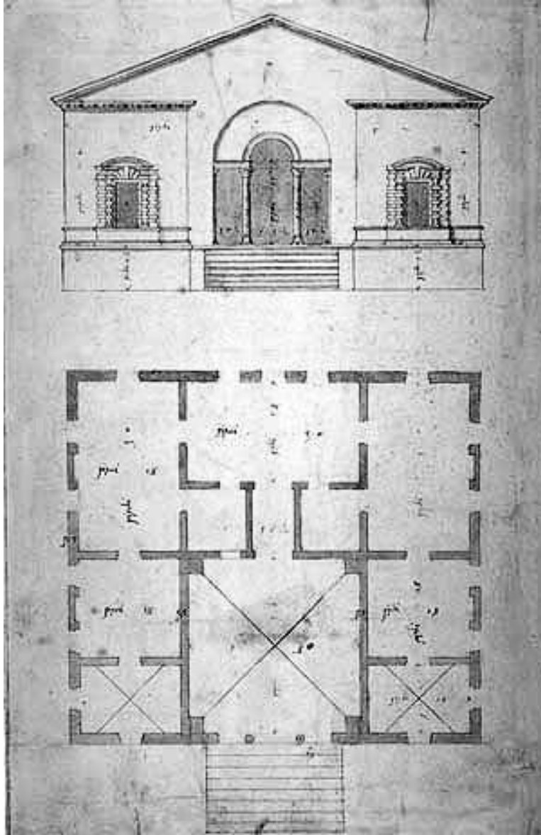
Вилла Вальмарана близ Виченцы, 1542 г., архитектор Андреа Палладио
