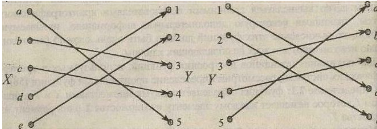
Рис. 1. Биективная функция f и обратная к ней g=f^{-1}
